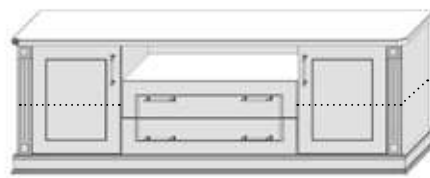
Yv.TTV.0-1 □ 1684 □ 575 □ 490
