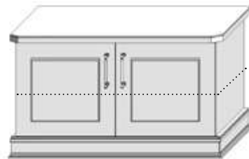
Yv.TPR-N2 □ 806 □ 461 □ 430
